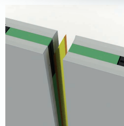
Jonction panneau étanche Airtight panel junction
